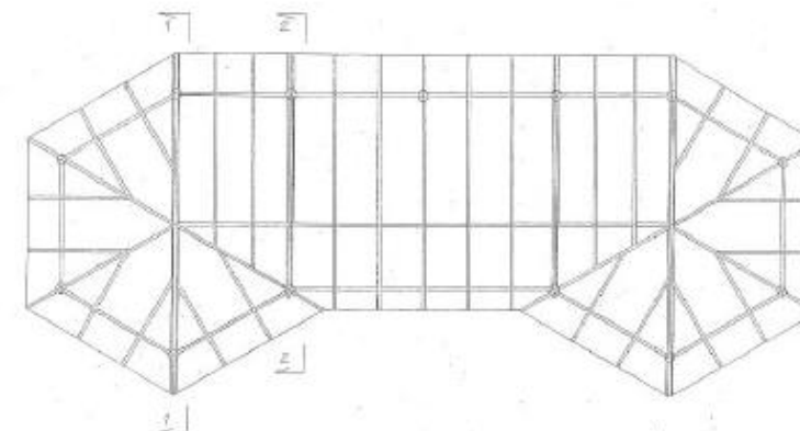
Vorlegeplan (Draufsicht)
